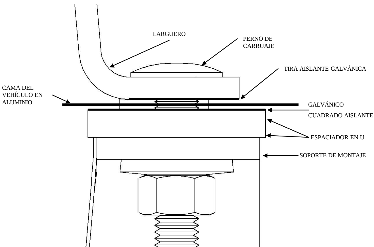
Figura 4: Tira aislante en el espaciador en forma de U
