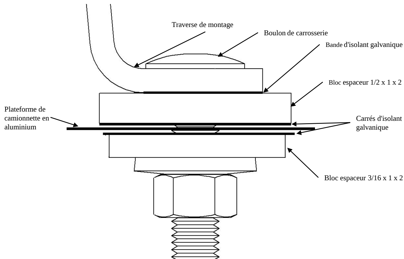
Figure 5 – Bandes d'isolant sur espaceurs pour boulons de traverse centrale
